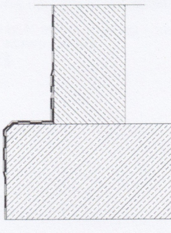
Bild A.5 — Anschluss Bodenfeuchte, Bitumenbahnen zweilagig versetzt verlegt
